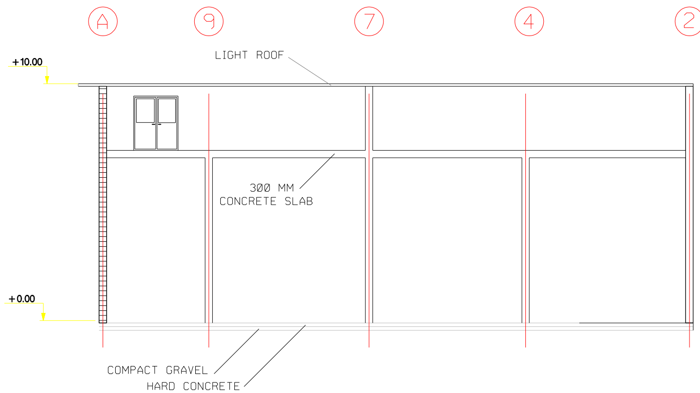
SECTION A-A
